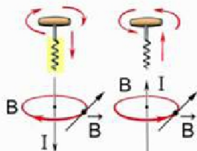
Правило буравчика
