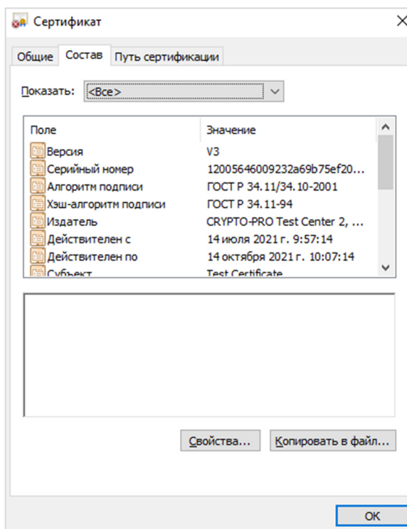
Рисунок 4. Вкладка «Состав»
